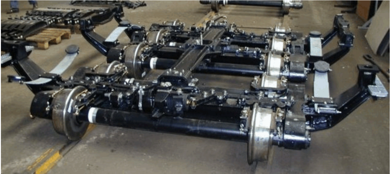
5-NÁPRAVOVÝ PODVOZOK RoLa
