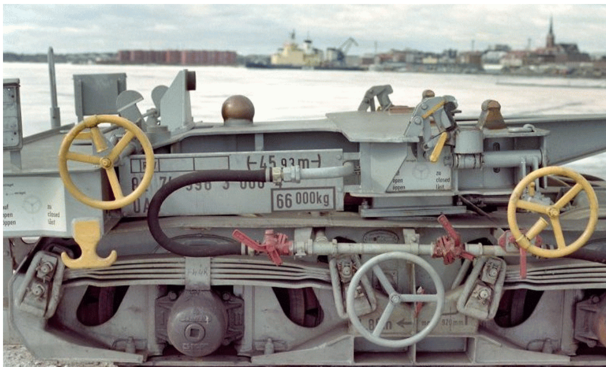
DETAIL PODVOZKU S KONCOVÝM ADAPTÉROM - SYSTÉM CODA-E
