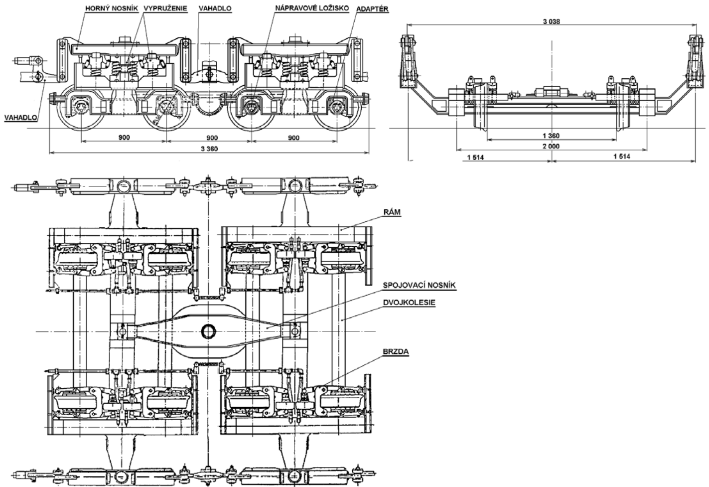
NÁČRTOK 4-NÁPRAVOVÉHO PODVOZKU RoLa
