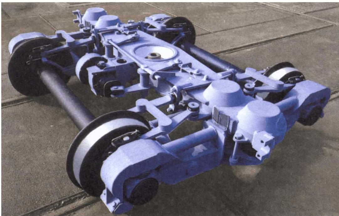
ČASŤ PODVOZKU RoLa (Talbot)
