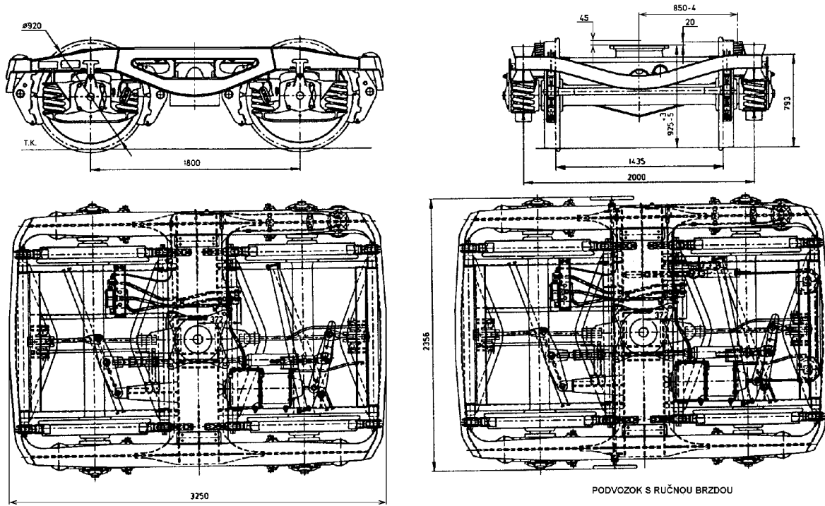
PODVOZOK Y 25 Ls(s)i1, Y 25 Ls(s)i1f (Tatravagónka, a.s. Poprad)
