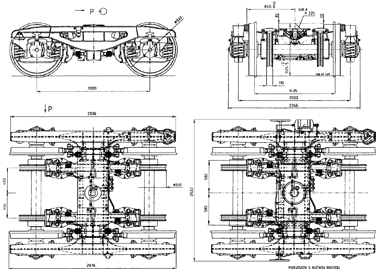
PODVOZOK Y 25 LasA (Tatravagónka a.s. Poprad)
