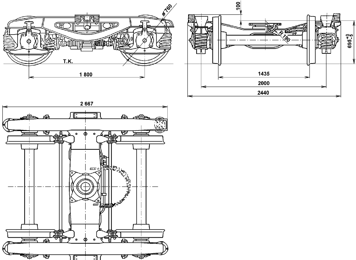
PODVOZOK Y 31 Lif (Tatravagónka a.s. Poprad)
