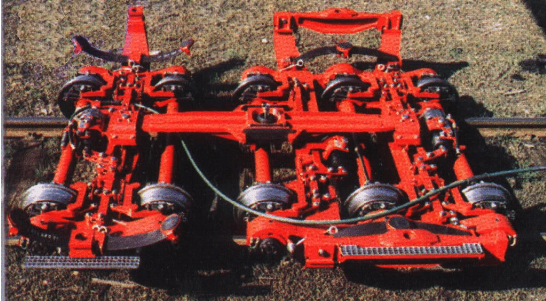
5-NÁPRAVOVÝ PODVOZOK RoLa
