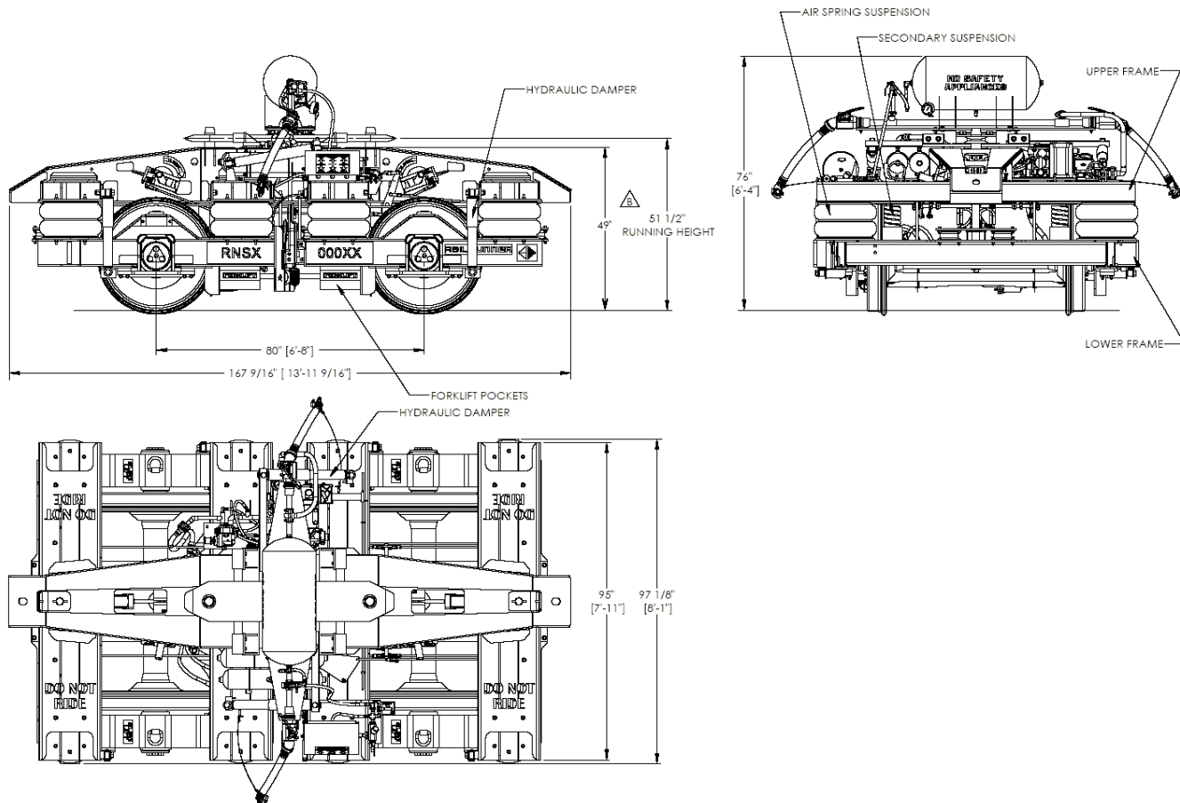
ROZMEROVÝ NÁČRTOK STREDOVÉHO PODVOZKU SYSTÉMU RailRunner (USA)
