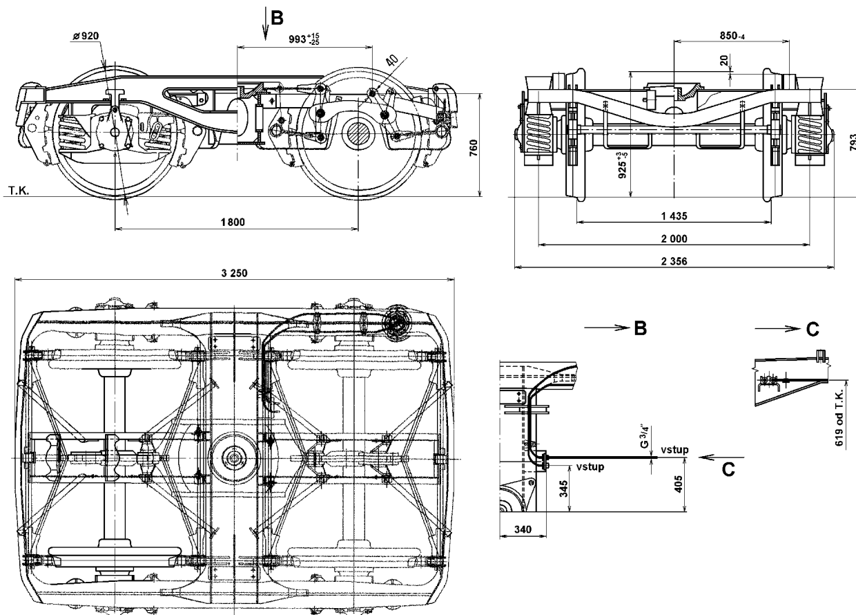
PODVOZOK Y 25 Ls(s)d1 (Tatragagónka, a.s. Poprad)
