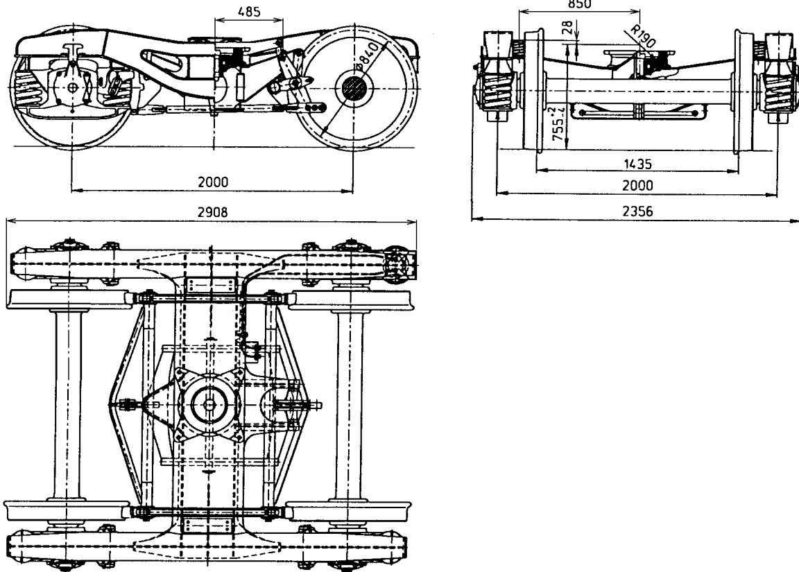
PODVOZOK Y 33 (Tatravagónka, a.s. Poprad)
