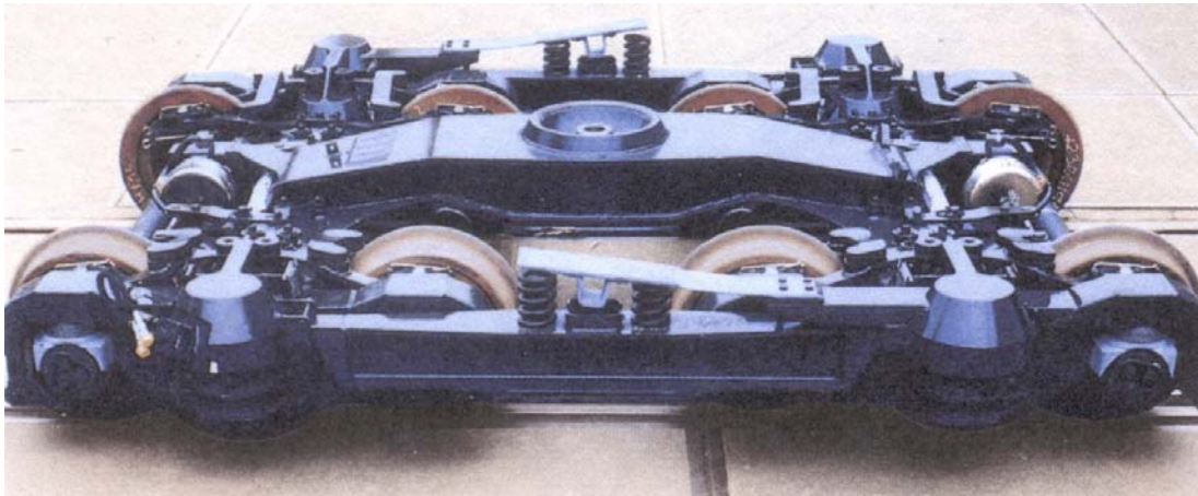
4-NÁPRAVOVÝ PODVOZOK RoLa (Talbot)
