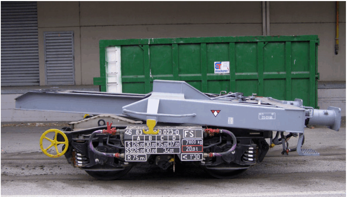
KONCOVÝ PODVOZOK PRE PREDNÉ ČELO NÁVESU SYSTÉMU Breda Carro Bimodale (Taliansko)
