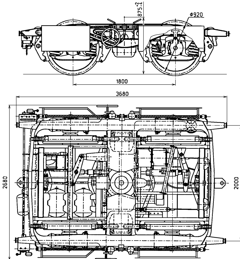
PODVOZOK Y 25-RRR PRE ROAD RAILER (Tatravagónka a.s. Poprad)
